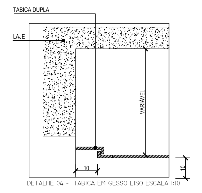
DETALHE TABICA EM GESSO LISO esc.: 1: 10
