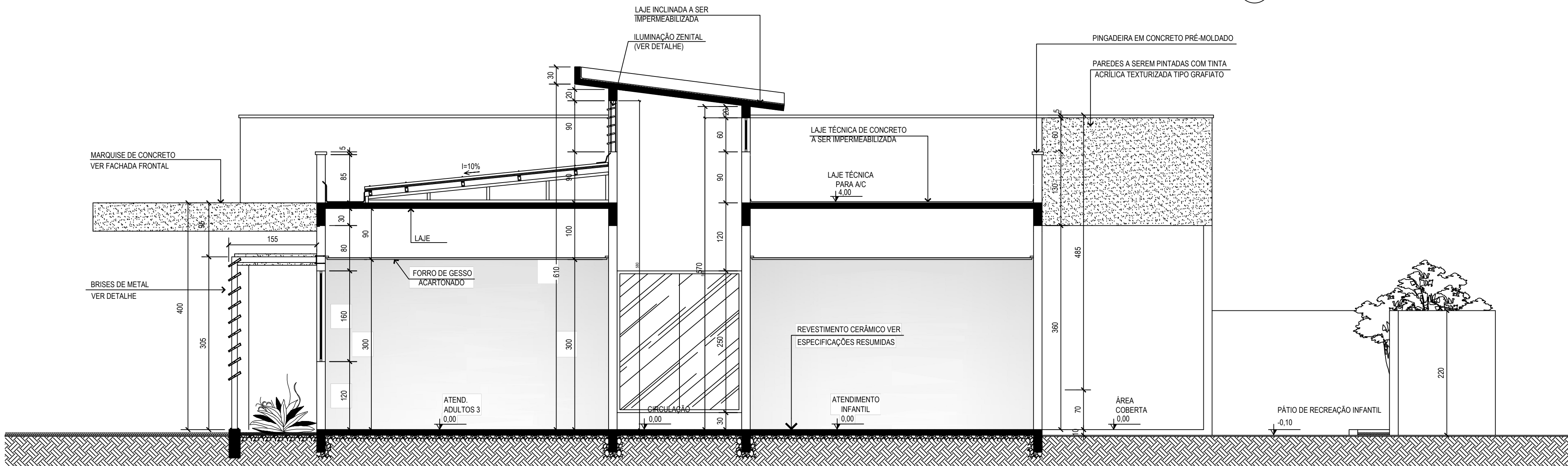
1 CORTE B-B esc.: 1: 50
