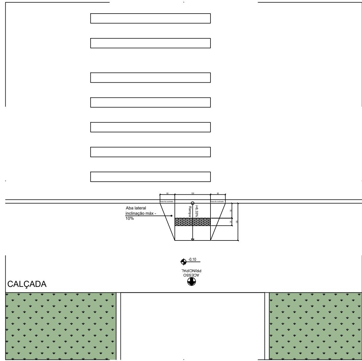
2 DET. REBAIXO DO MEIO FIO esc.: 1: 75
