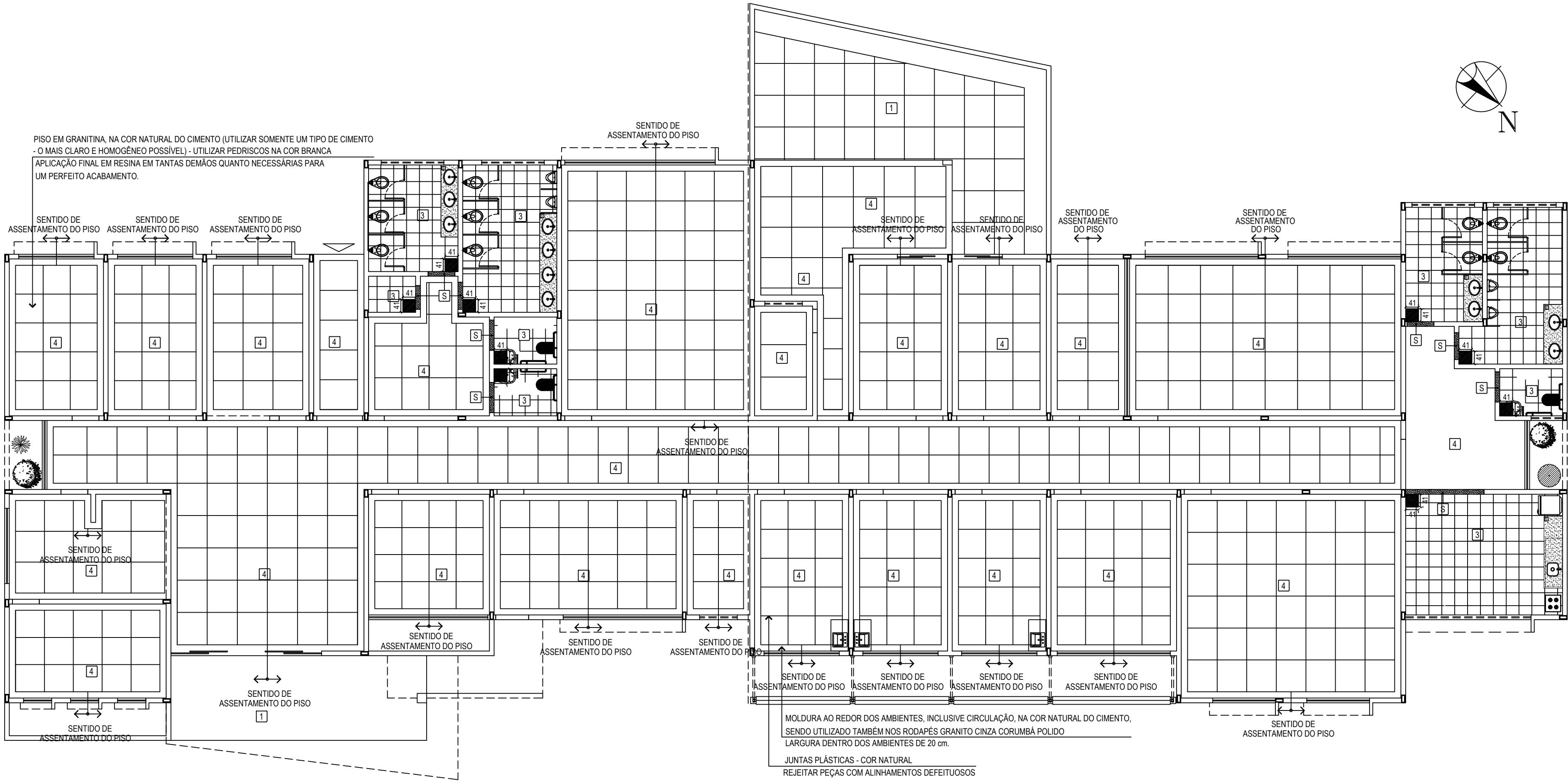
2 PLANTA DE PAGINAÇÃO INTERNA esc.: 1: 100
