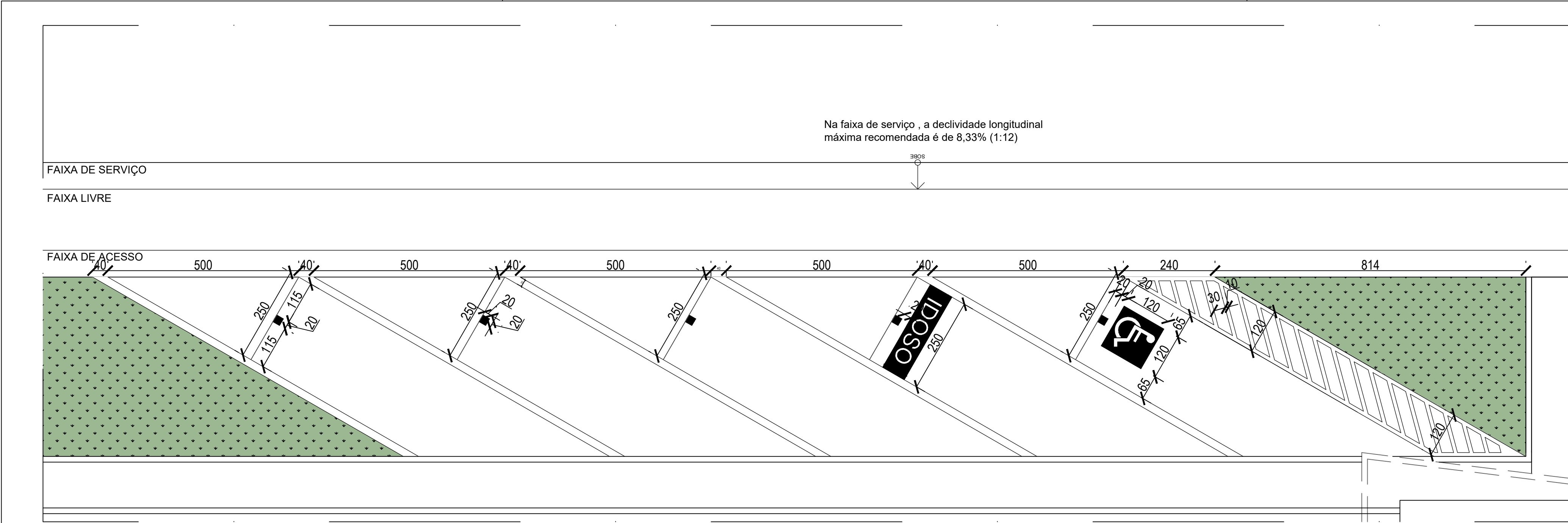
1 DET. ESTACIONAMENTO esc.: 1: 75
