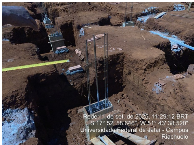
Forma dos pilaretes
