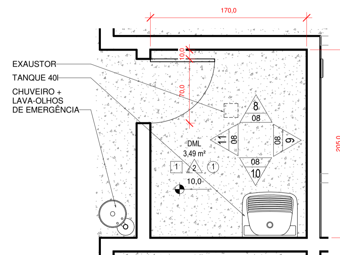
7 DETALHAMENTO - DML 1 : 25
