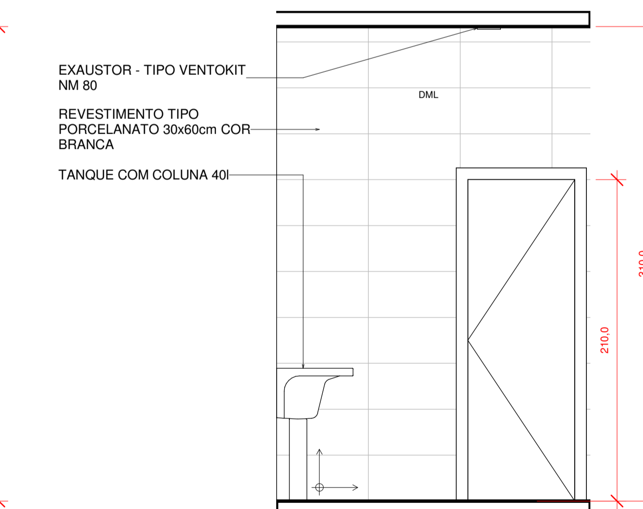
11 DML - PAREDE 4 1 : 25
