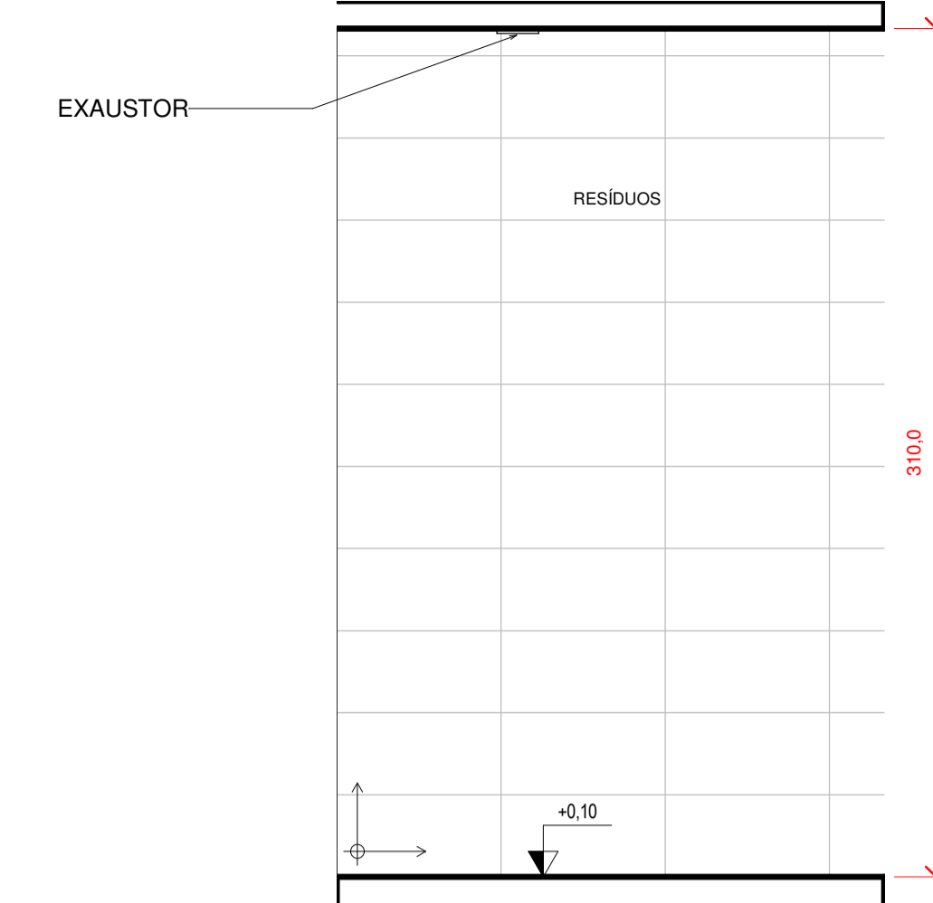
4 RESÍDUOS - PAREDE 2 1 : 25
