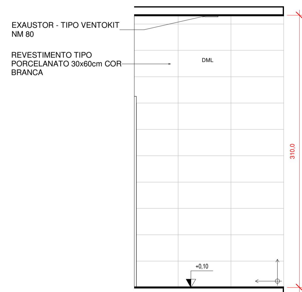
8 DML - PAREDE 1 1 : 25
