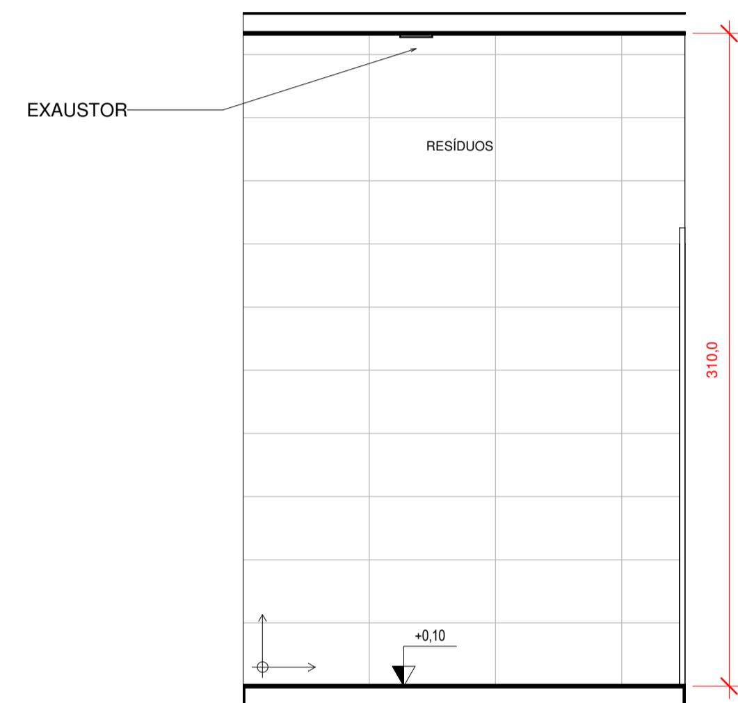
5 RESÍDUOS - PAREDE 3 1 : 25
