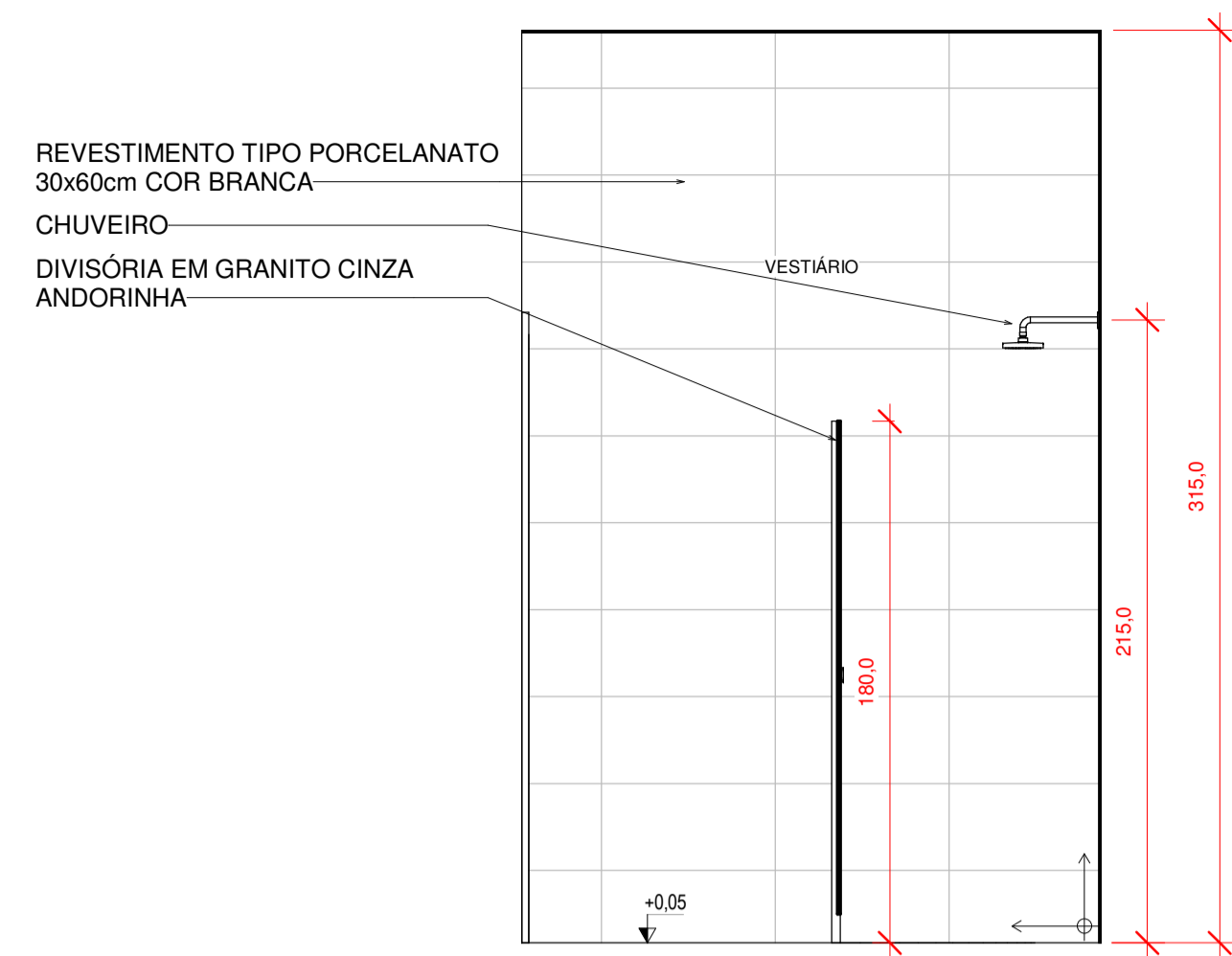
1 VESTIÁRIO - PAREDE 4 1 : 25
