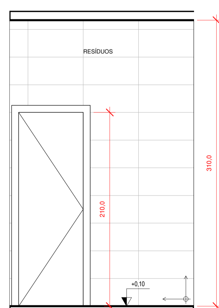
6 RESÍDUOS - PAREDE 4 1 : 25
