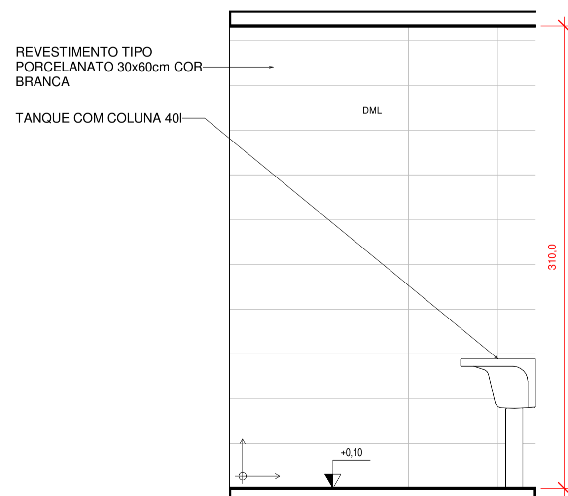
9 DML - PAREDE 2 1 : 25
