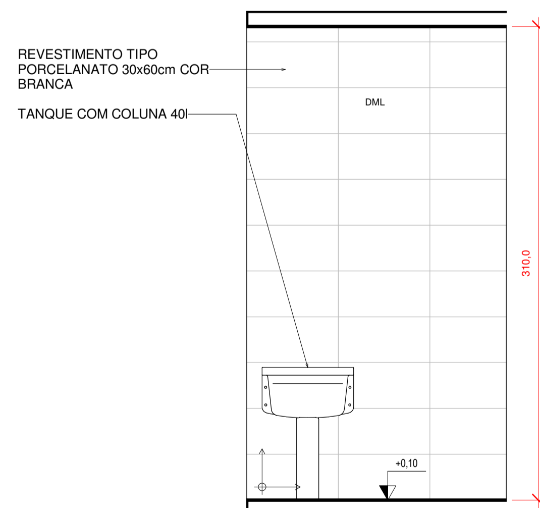
10 DML - PAREDE 3 1 : 25
