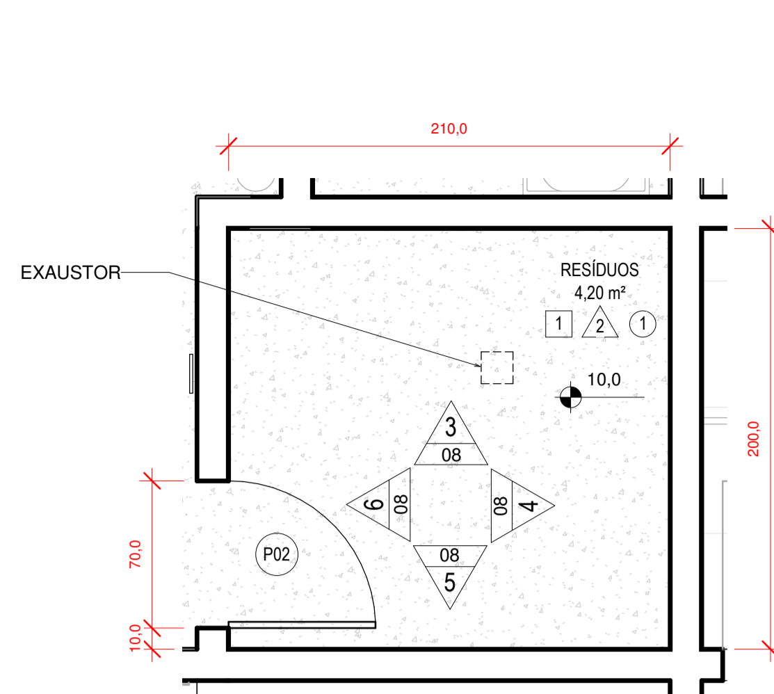
2 DETALHAMENTO - RESÍDUOS 1 : 25
