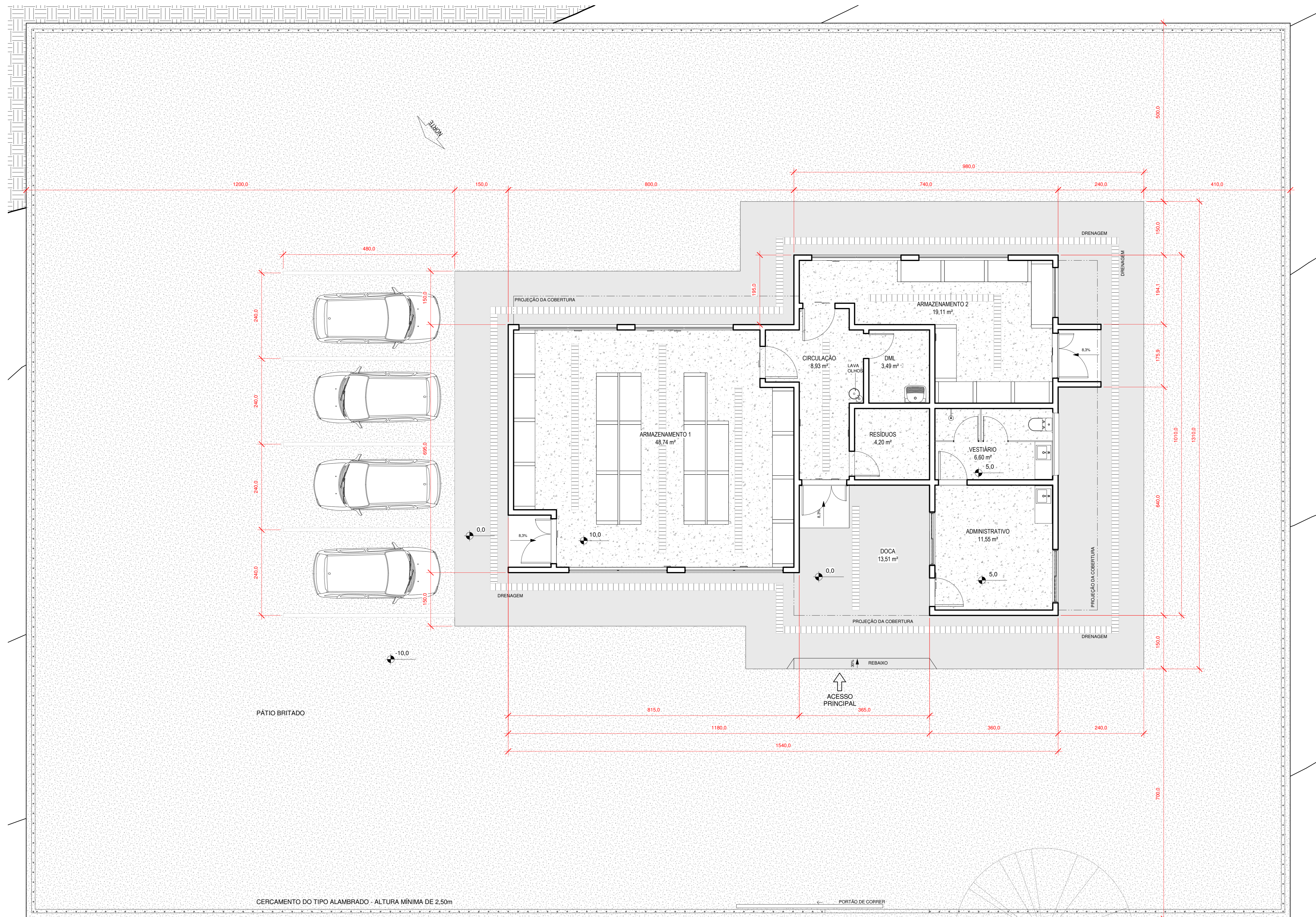
1 PLANTA BAIXA GERAL 1 : 50
