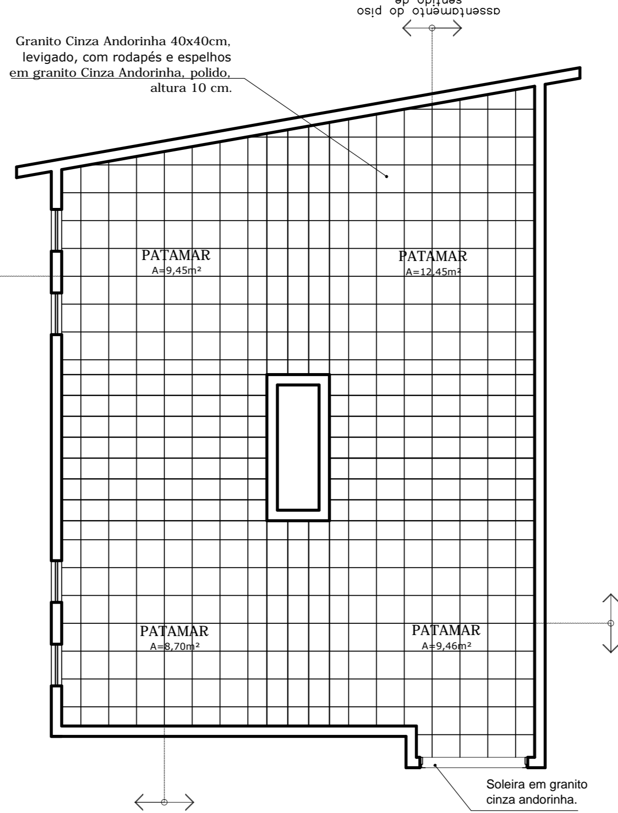
Detalhe paginação da escada esc.1:50
