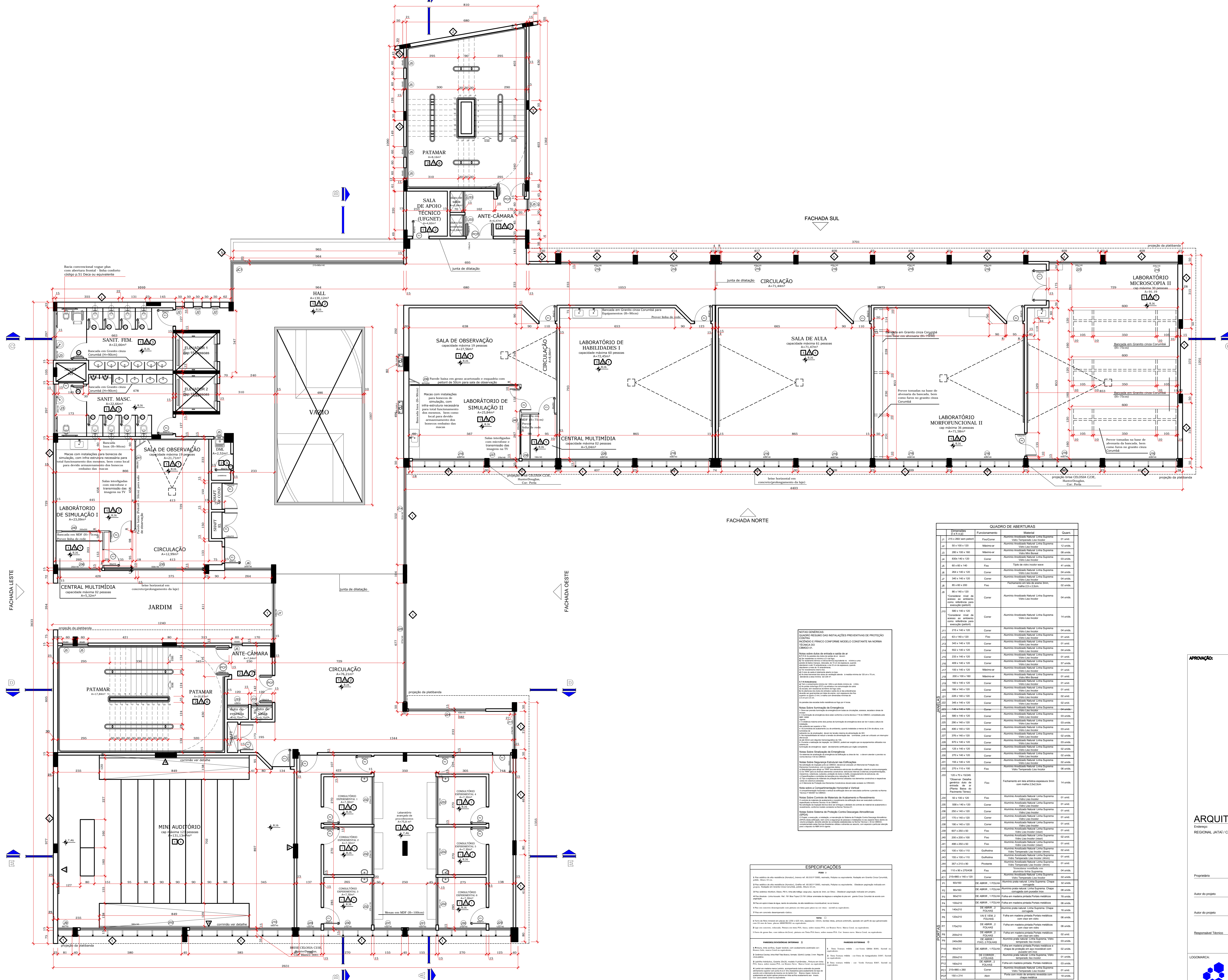
PLANTA BAIXA - SEGUNDO PAVIMENTO esc.1:75
