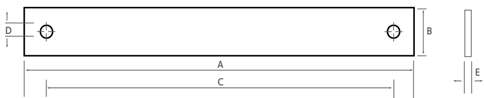
(A) Comprimento total (mm) (B) Largura (C) Distância entre centros de furos (mm) (D) Diâmetro dos furos (E) Espessura
