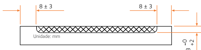
Desenho Barra Chata Esteira em corte transversal
